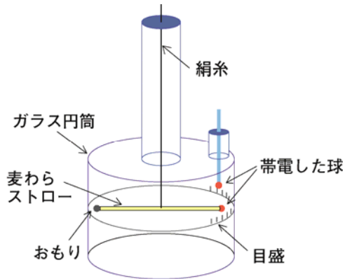
図 9 クーロンの秤
